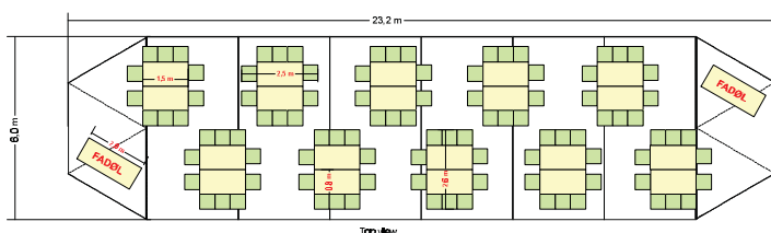
Perspektiv tegning af 18 x 6 m. telt med 2 x Apsis grå/hvid alt ca. 138 m 2
